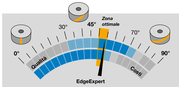
Leitz EdgeExpert: angolo di taglio regolato in modo ottimale
